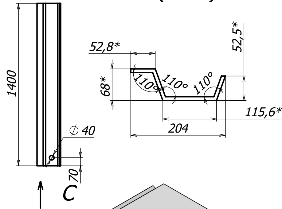
C (1 : 5)
